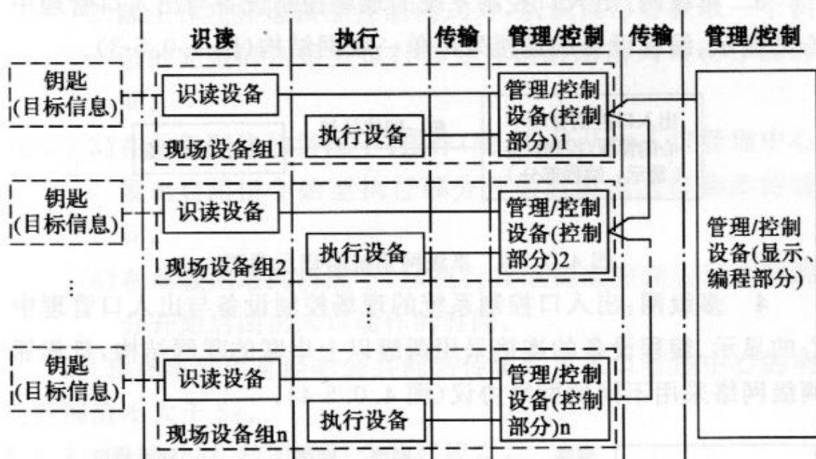
图 4.0.5-1 总线制系统组成
