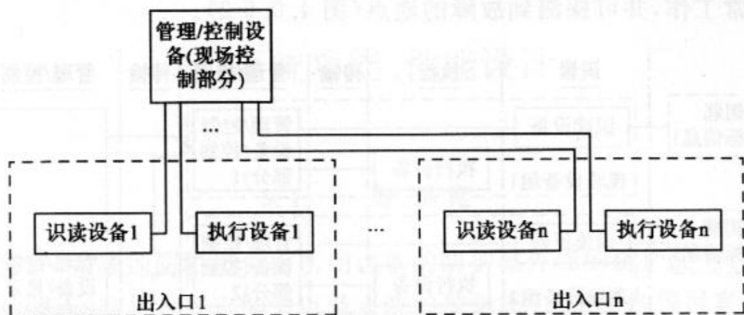
图 4.0.4-2 多出入口控制设备型组成
