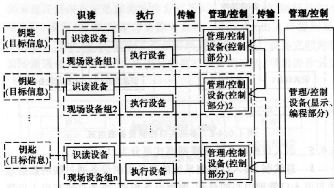
图 4.0.5-2 环线制系统组成
