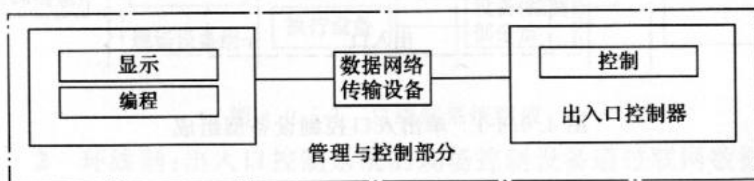
图 4.0.3-2 联网控制型组成
